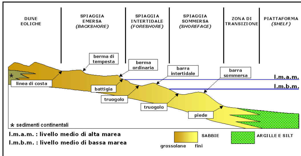
Figura 1: Profilo geomorfologico ideale schematico (non in scala) di una spiaggia (immagine tratta da Wikipedia).
